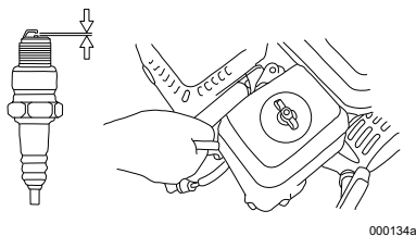
Figure 4-10. Bougie d'allumage
